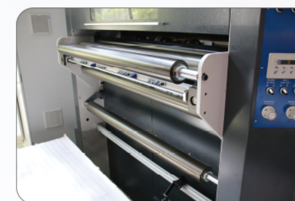
电动小反曲控制系统 Electric de-curl unit
