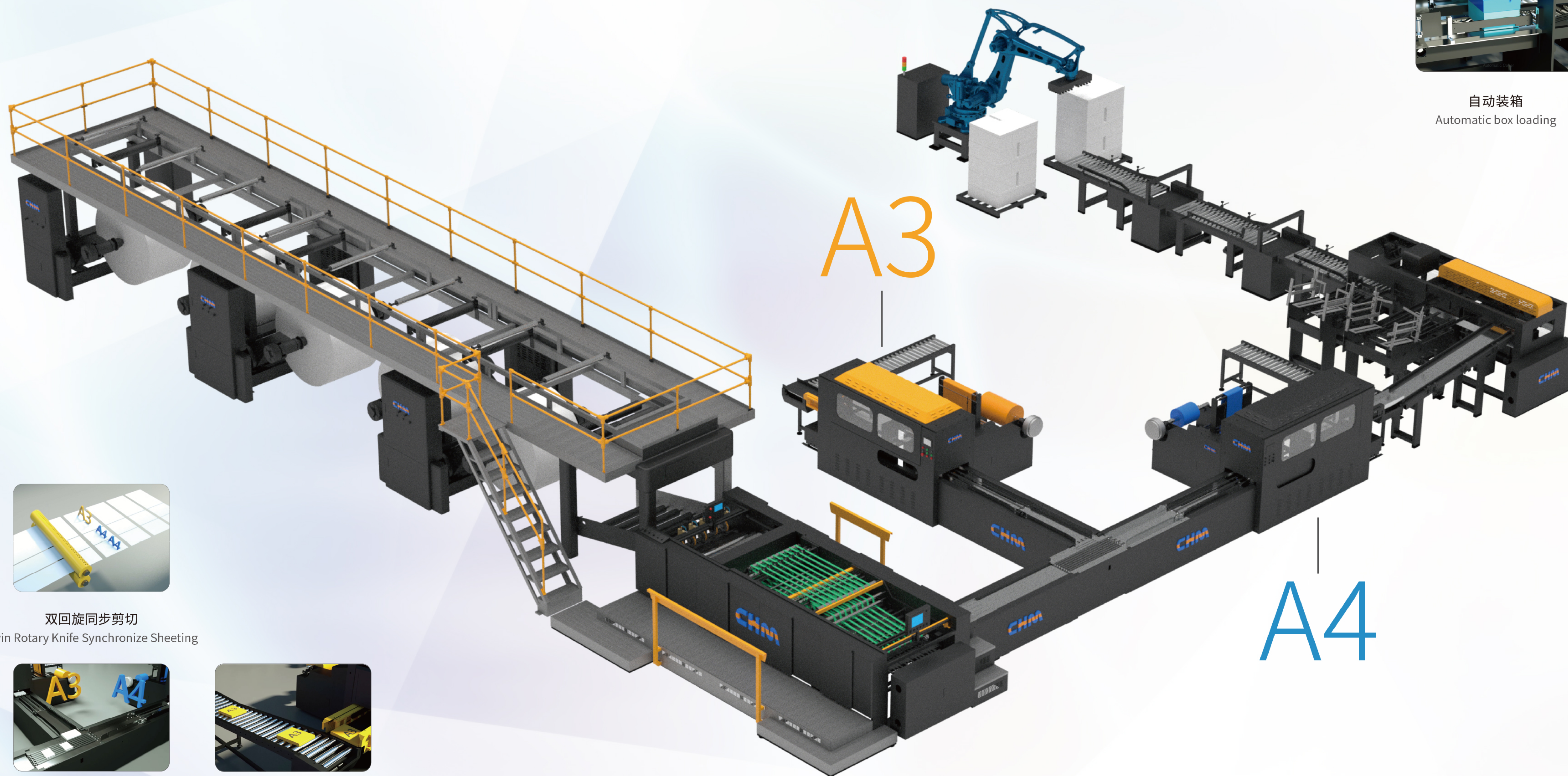
令纸输送 Ream output
